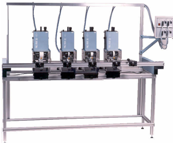
Mehrkopfanlage mit Einlegeschlitten für Ring- und Textbedruckung
